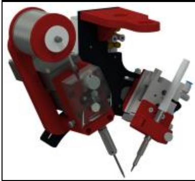
SH5500I_P_ Roboterlötkopf mit Pneumatischem Zylinder / Reinigungsstation / Drahtjustierereinheit / Kabellänge 5m Robotic soldering head with pneumatic cylinder / Tip cleaner / Wire adjustment unit / Cable 5m
